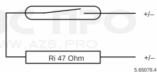
Схема подключения RV
