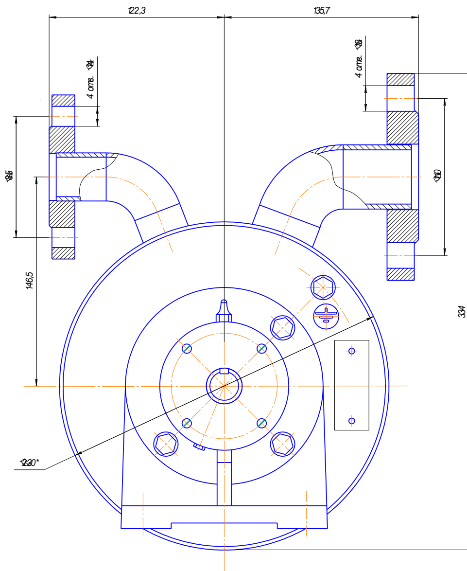
рисунок 2а. Насос
